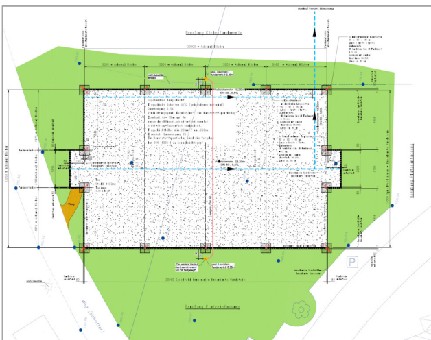
Ausschnitt Lageplan
